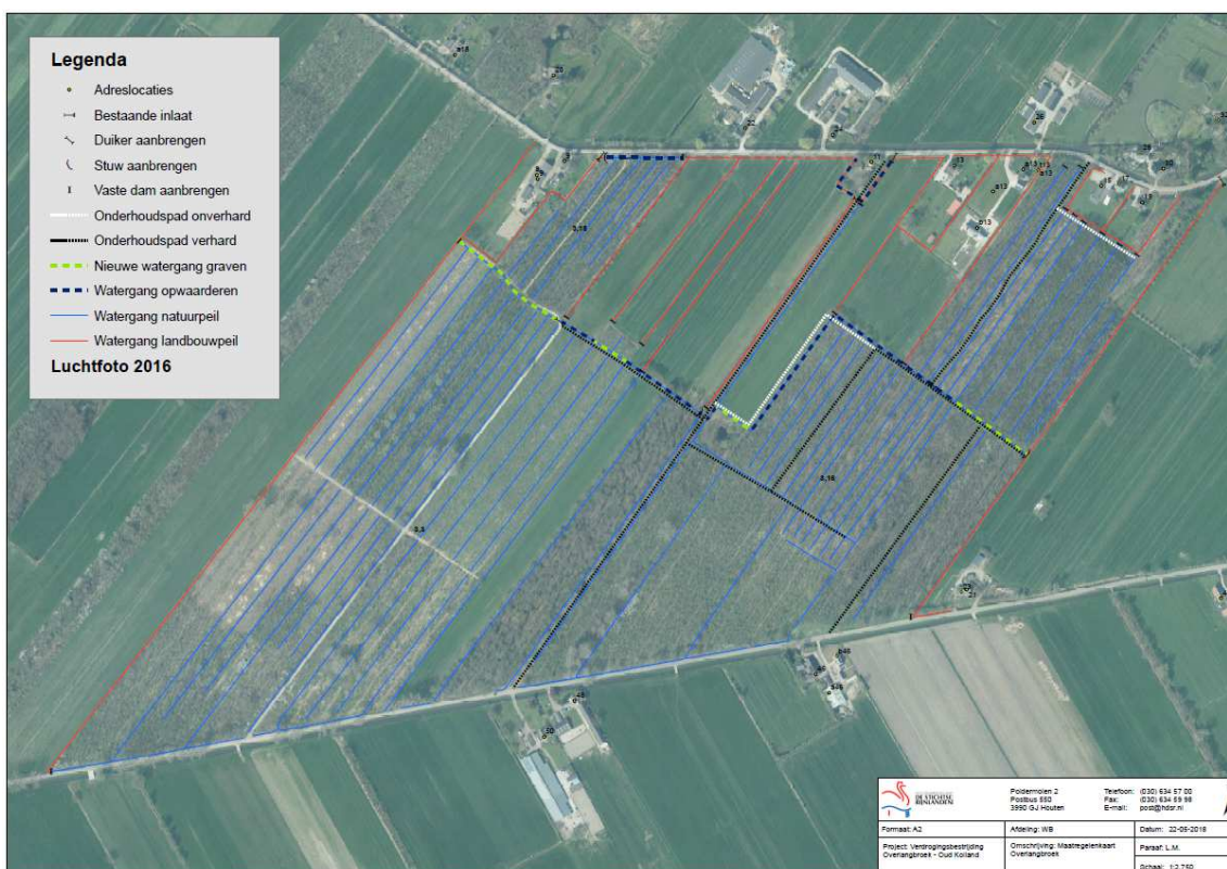
Figuur 2. Inrichtingsplan / uit te voeren maatregelen
