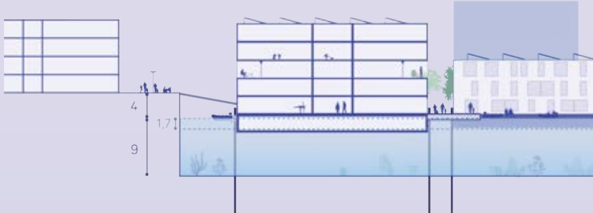
Doorsnede C
