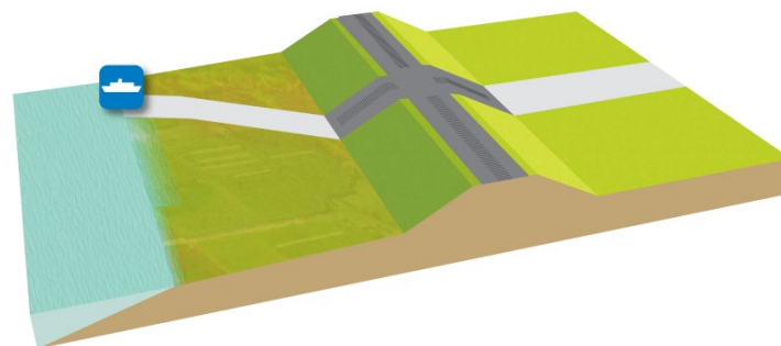
01. Principeschema dijkopgang landelijk gebied (basisprofiel tot omliggende maavelde)
