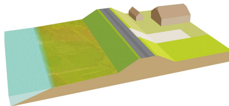
03. Principeschema dijkopgang erf-inritten (aansluiting erf op basisprofiel)
