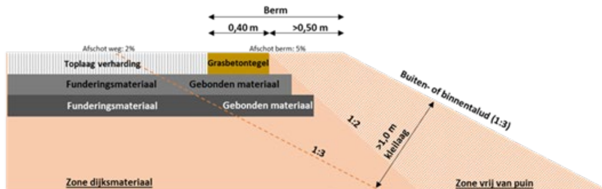
Standaardontwerp wegberm op een dijk
