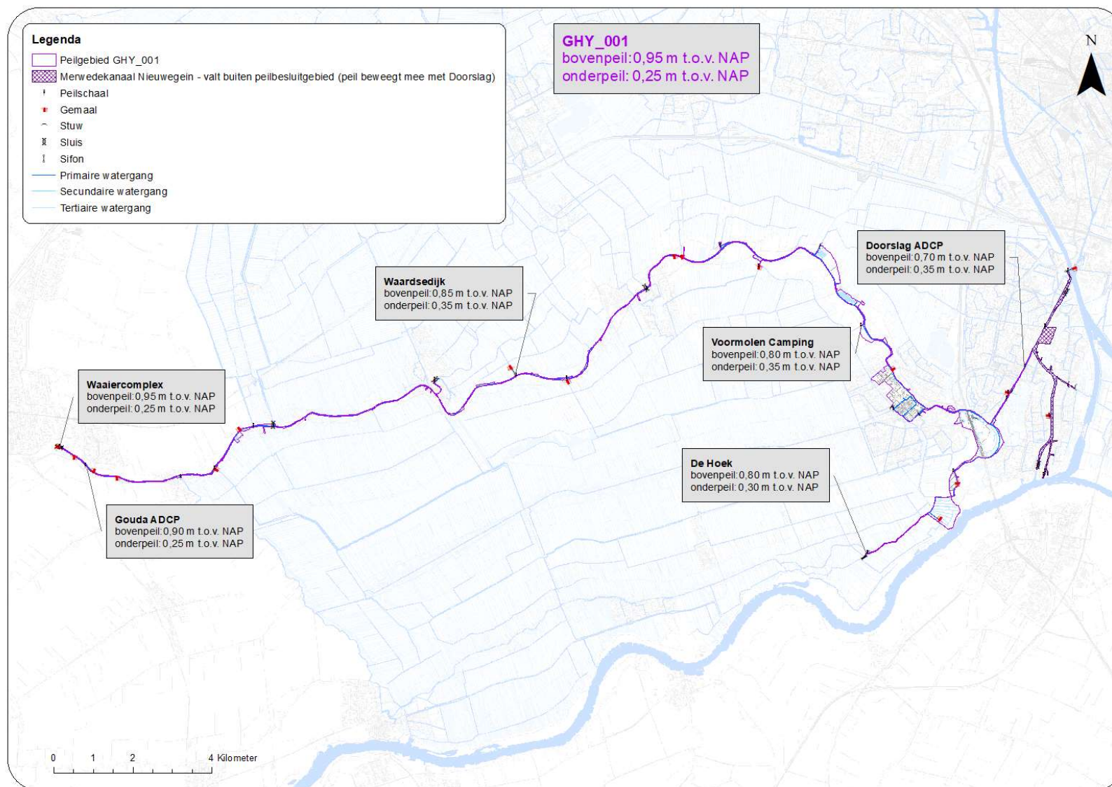
Figuur 14: Overzicht boven- en onderpeilen (in m t.o.v. NAP) langs het boezemwatersysteem van de GHJ. In het paars het absolute boven- en onderpeil.
