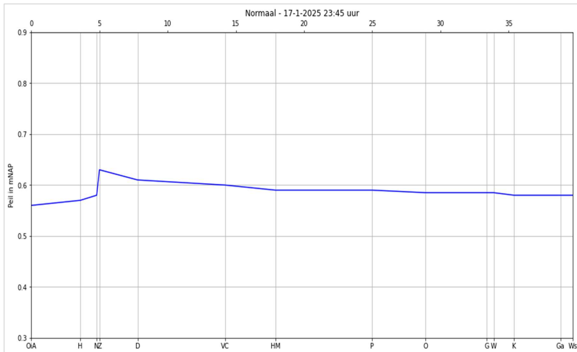
Figuur 8: Indicatie van de verhanglijn in een normale situatie. De grafiek weergeeft waterhoogtemetingen van 17 januari 2025 om 23:45 uur op de locaties Oog in Al (OIA), Hoograven (H), Noordergemaal (N), Zuidersluis (Z), Doorslag (D), Voormolen Camping (VC), Hoekse molen (HM), Pleyt (P), Sluis Oudewater (O), Goejanverwellesluis (G), Wiericksoord (W), Keulevaart (K), Gouda (Ga) en Waaiersluis (Ws). Ten behoeve van de leesbaarheid en correctheid van de verhanglijn zijn er handmatige correcties gedaan ten opzichte van de ruwe meetgegevens.
