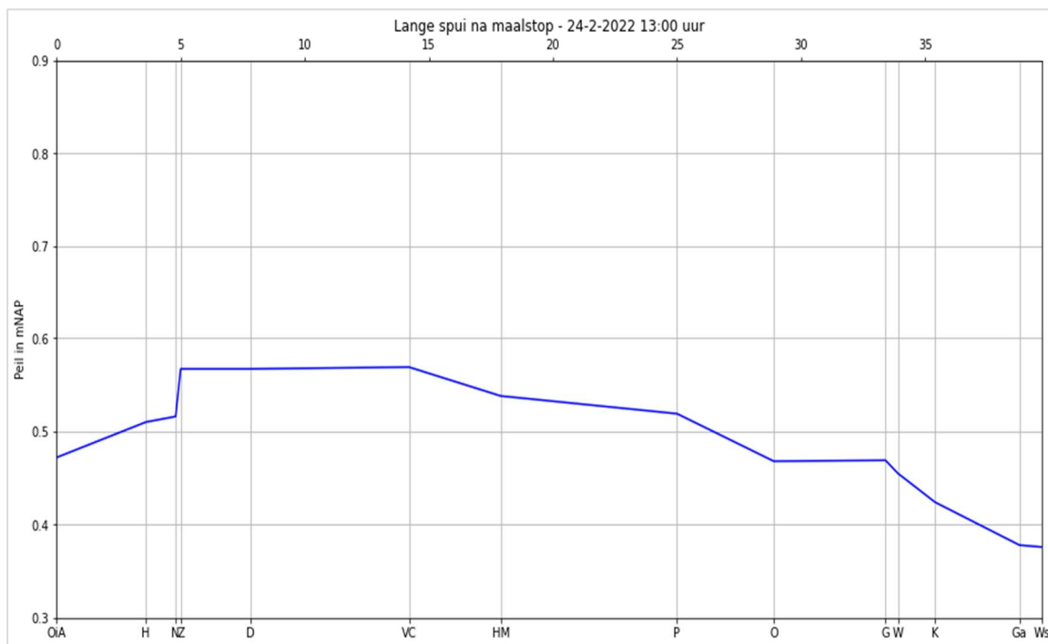
Figuur 9: Indicatie van de verhanglijn in een natte situatie waarbij langere tijd gespuid wordt na een maalstop. De grafiek weergeeft waterhoogtemetingen van 24 februari 2022 om 13:00 uur op de locaties Oog in Al (OIA), Hoograven (H), Noordergemaal (N), Zuidersluis (Z), Doorslag (D), Voormolen Camping (VC), Hoekse molen (HM), Pleyt (P), Sluis Oudewater (O), Goejanverwellesluis (G), Wiericksoord (W), Keulevaart (K), Gouda (Ga) en Waaiersluis (Ws). Ten behoeve van de leesbaarheid en correctheid van de verhanglijn zijn er handmatige correcties gedaan ten opzichte van de ruwe meetgegevens.
