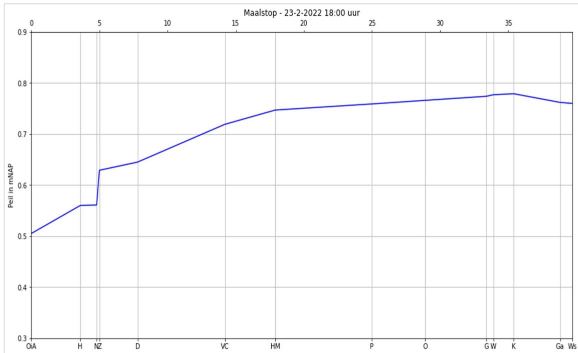
Figuur 10: Indicatie van de verhanglijn in een natte situatie waarbij een maalstop geldt voor de poldergemalen. De grafiek weergeeft waterhoogtemetingen van 23 februari 2022 om 18:00 uur op de locaties Oog in Al (OiA), Hoograven (H), Noordergemaal (N), Zuidersluis (Z), Doorslag (D), Voormolen Camping (VC), Hoekse molen (HM), Pleyt (P), Sluis Oudewater (O), Goejanverwellesluis (G), Wiericksoord (W), Keulevaart (K), Gouda (Ga) en Waaiersluis (Ws). Ten behoeve van de leesbaarheid en correctheid van de verhanglijn zijn er handmatige correcties gedaan ten opzichte van de ruwe meetgegevens.
