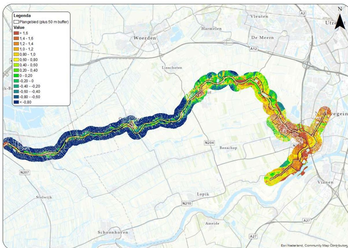
Figuur 17: Maaiveldhoogtekaart. Voor het berekenen van de maaiveldhoogte is gebruik gemaakt van het meest recente Actueel Hoogtebestand Nederland, het AHN5. De grens van het plangebied valt binnen de zwarte lijnen.
