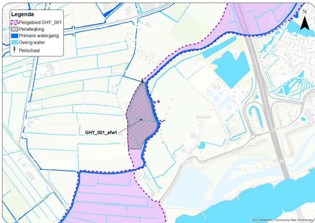
Figuur 16: De peilafwijking in het plangebied: onderbemaling aan de Lage Dijk-Zuid.
