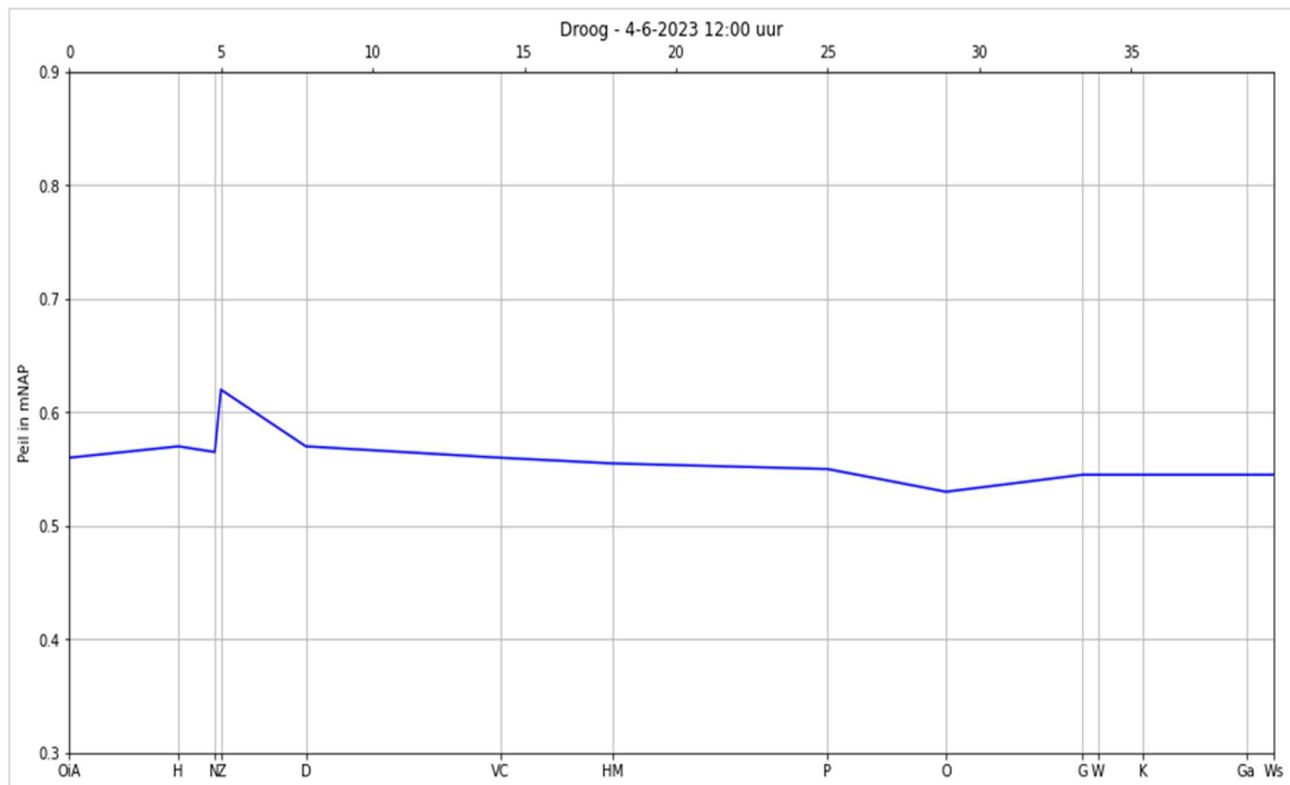
Figuur 11: Indicatie van de verhanglijn in een droge situatie. De grafiek weergeeft waterhoogtemetingen van 4 juni 2023 om 12:00 uur op de locaties Oog in Al (OIA), Hoograven (H), Noordergemaal (N), Zuiderluis (Z), Doorslag (D), Voormolen Camping (VC), Hoekse molen (HM), Pleyt (P), Sluis Oudewater (O), Goejanvervellesluis (G), Wiericksoord (W), Keulevaart (K), Gouda (Ga) en Waaiersluis (Ws). Ten behoeve van de leesbaarheid en correctheid van de verhanglijn zijn er handmatige correcties gedaan ten opzichte van de ruwe meetgegevens.
