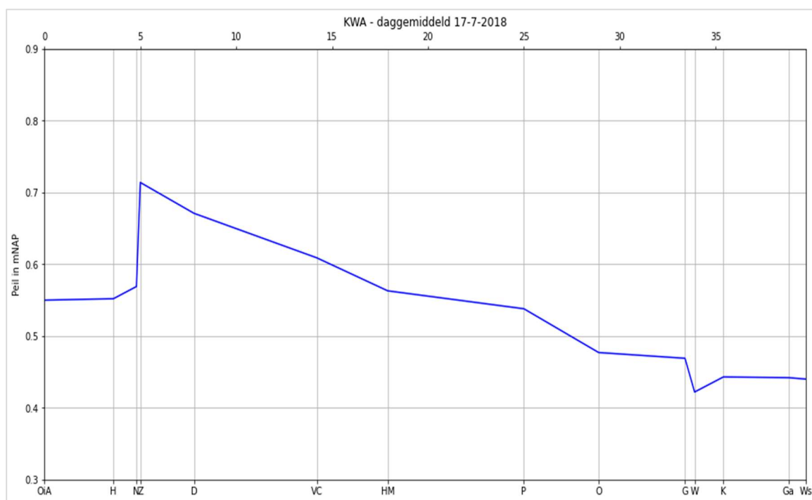
Figuur 12: Indicatie van de verhanglijn in een KWA- situatie. De grafiek weergeeft waterhoogtemetingen van 17 juli 2018 op de locaties Oog in Al (OIA), Hoograven (H), Noordergemaal (N), Zuidersluis (Z), Doorslag (D), Voormolen Camping (VC), Hoekse molen (HM), Pleyt (P), Sluis Oudewater (O), Goejanverwellesluis (G), Wiericksoord (W), Keulevaart (K), Gouda (Ga) en Waaiersluis (Ws). Ten behoeve van de leesbaarheid en correctheid van de verhanglijn zijn er handmatige correcties gedaan ten opzichte van de ruwe meetgegevens.
