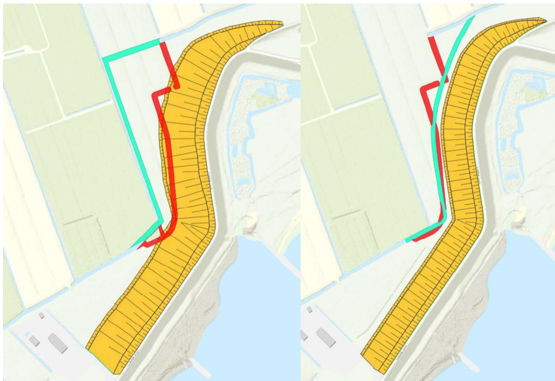
Figuur 2.2 Stabiliteitsberm De Drie Wielen in het ontwerp Projectbesluit (links) en het definitieve Projectbesluit (rechts), inclusief het dempen (rood) en opnieuw aanbrengen (groen) van de watergang
