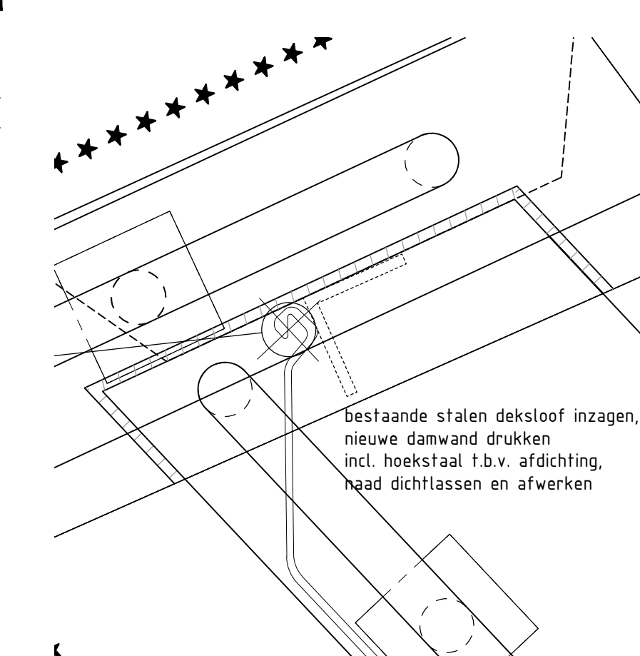
Detail aansluiting op damwand hoogwaterstuw schaal 1:5
