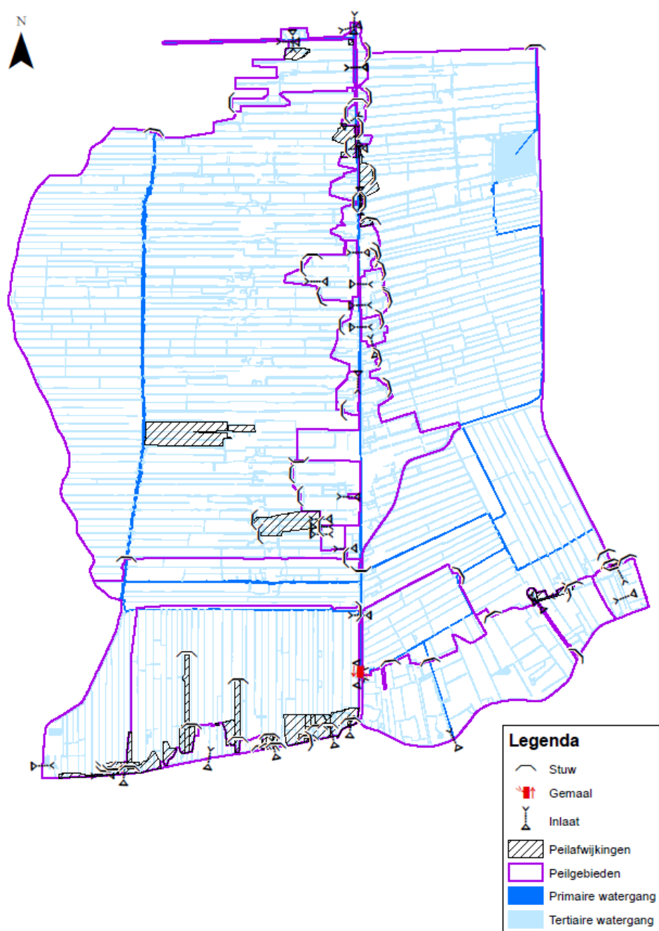
Figuur 6 Watersysteem
