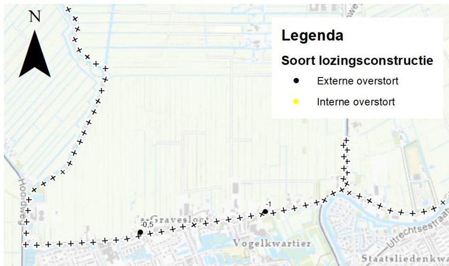
Figuur 9 Lozingspunten in het zuiden van het plangebied. De cijfers geven de hoogte van de overstordrempels aan in m t.o.v. NAP
