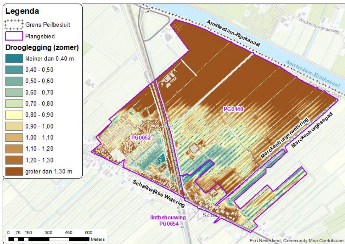
Figuur 15 Droogleggingskaart bij het zomerpeil (de ophoging van de woningbouwlocatie is nog niet meegenomen in de berekening van de drooglegging)
