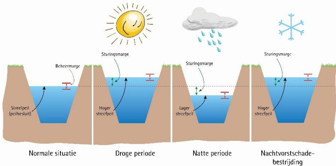
Figuur 12 Toepassen van sturingsmarge in het peilbeheer
