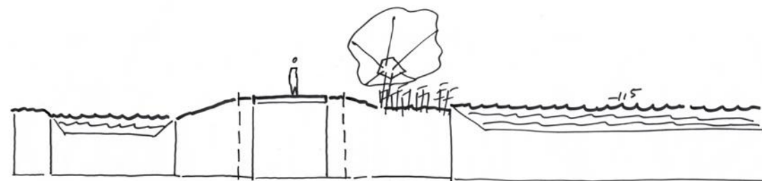
Typend profiel met de lage kade en de smalle oever
