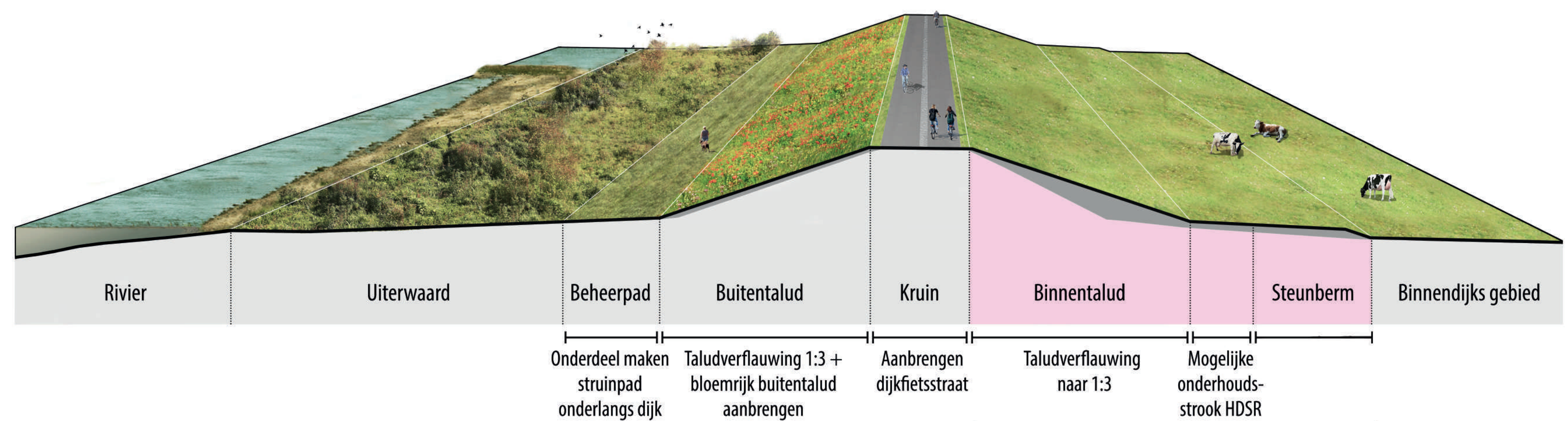
Ruimtelijke weergave van dijkmaatregelen tussen oostgrens en dijkpaal 91.
