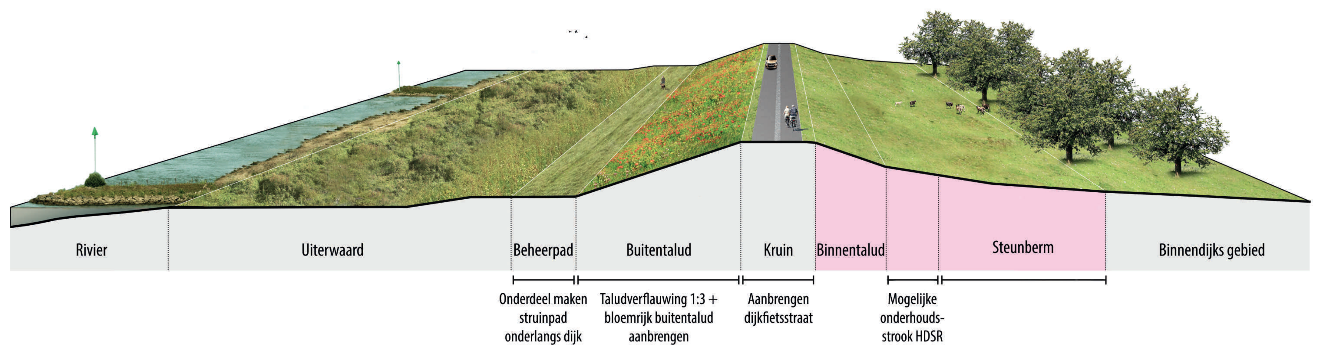
Ruimtelijke weergave van dijkmaatregelen tussen dijkpaal 91 en dijkpaal 95,5.
