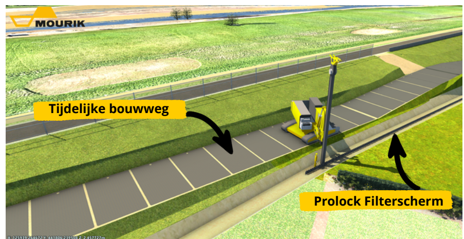
Afbeelding 1 - Impressie aanbrengen Prolock Filterscherm
