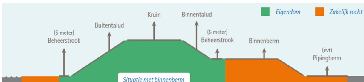
Figuur 3.1 Verwervingsstrategie met binnenberm
