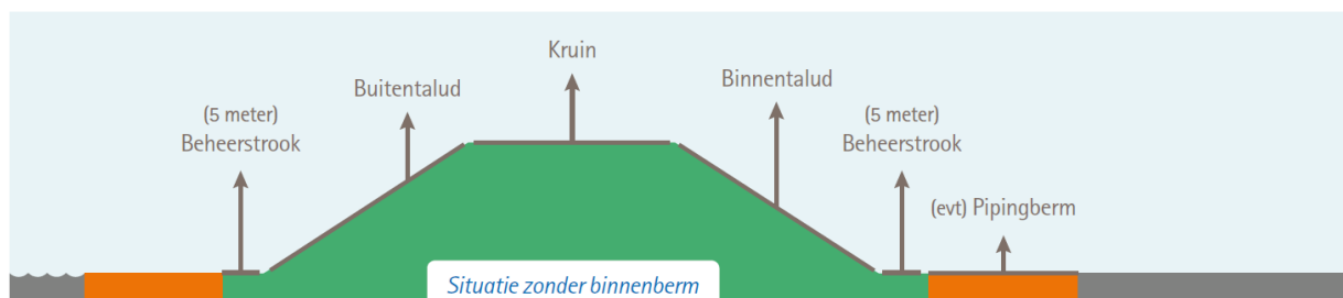
Figuur 3.2 Verwervingsstrategie zonder binnenberm
